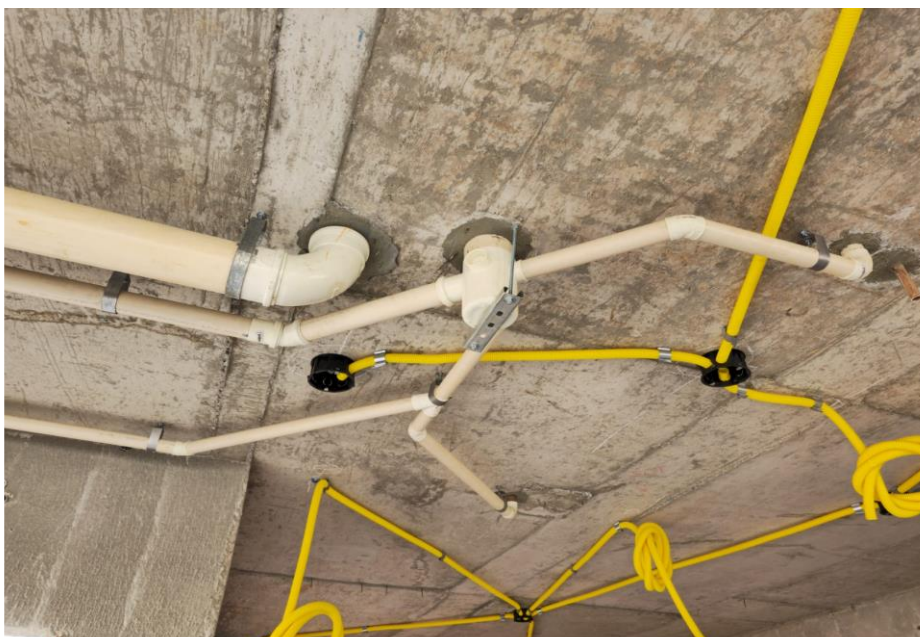
Infra de hidráulica e elétrica do 5º pavimento – Setembro 2024
