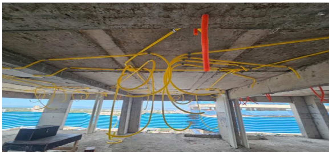
Instalações elétricas de teto até o 23º pavimento da Torre Parque – Junho 2026
