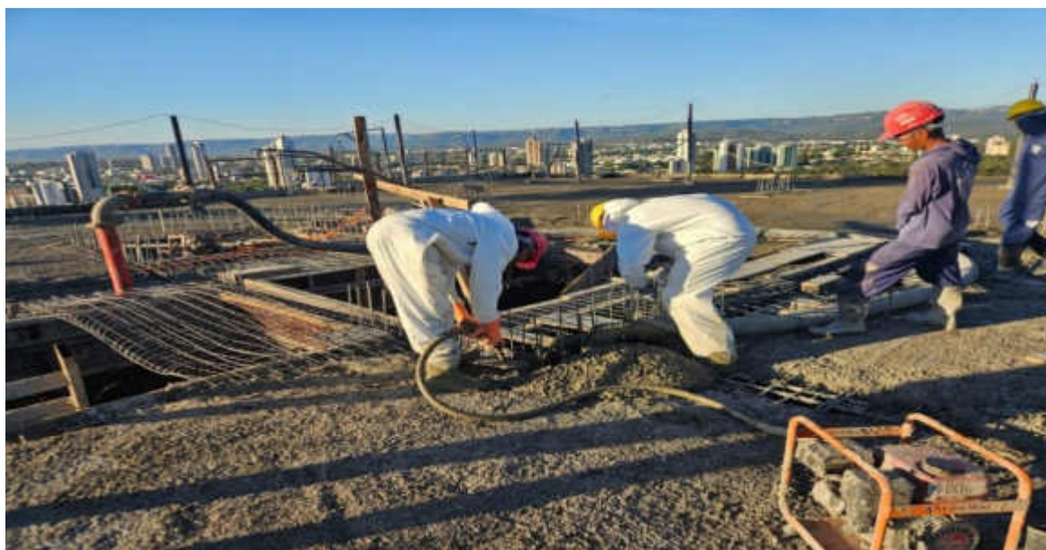
Estrutura do 33º pavimento da Torre Parque – Julho 2026
