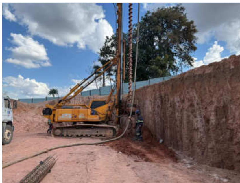
Execução de estaca hélice contínua (contenção - Rua Araxá) – Julho 2026
